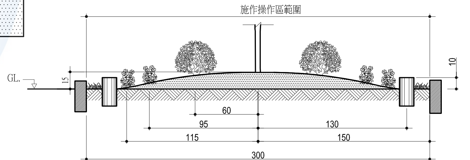
剖面圖 ② S=1 / 20
