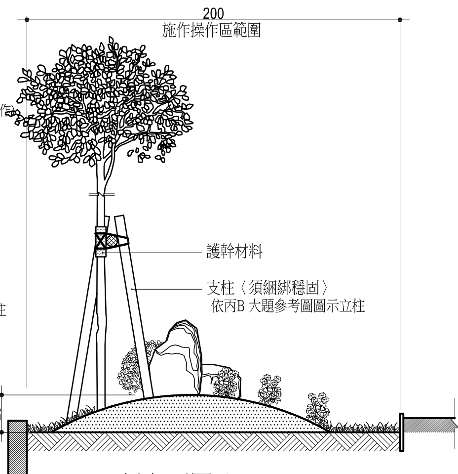
剖面圖 ① S=1 / 20
