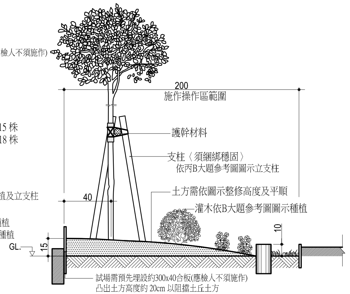
剖面圖 ① S=1 / 20
