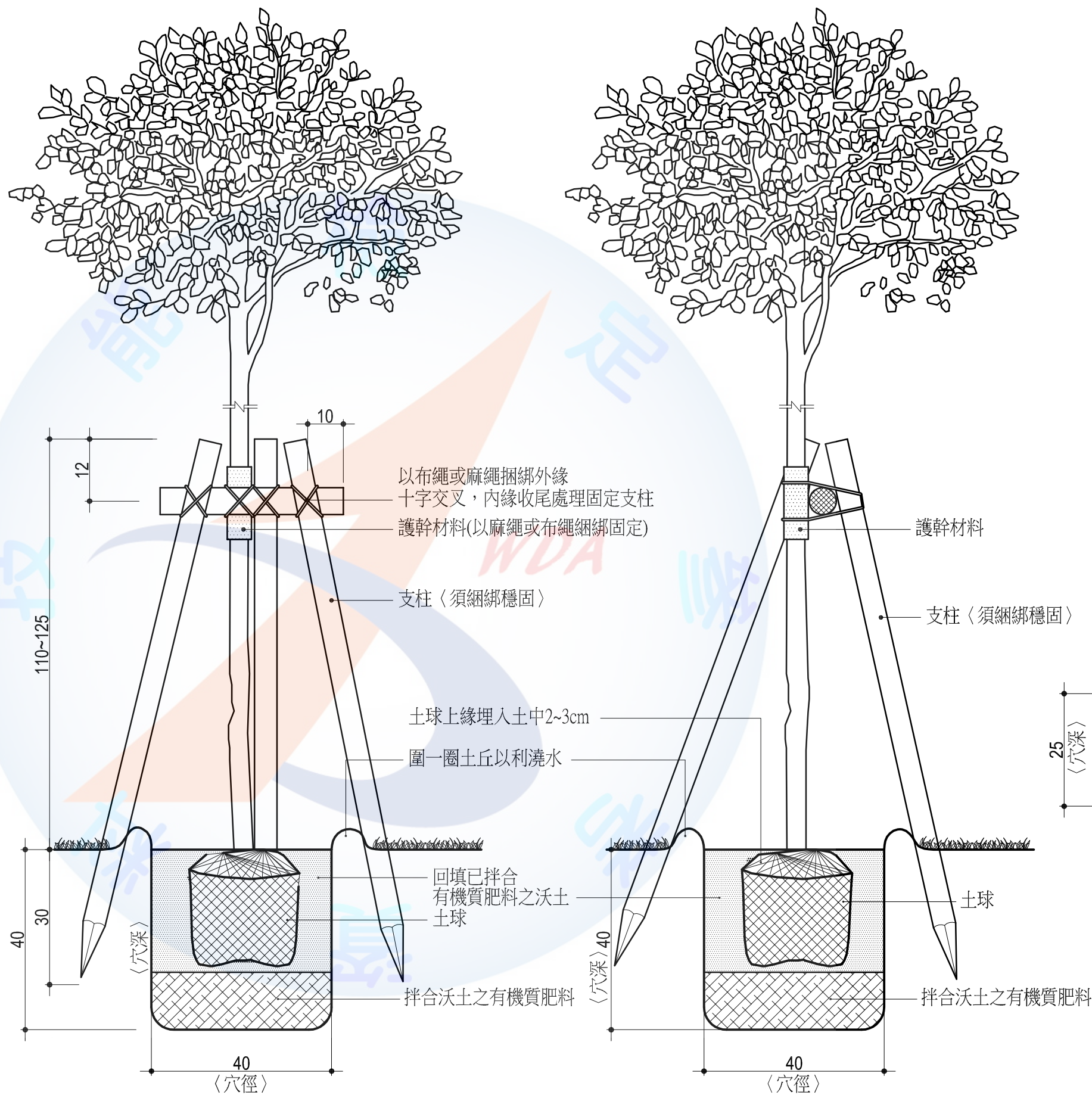
喬木栽植剖面示意圖S=1 / 10
