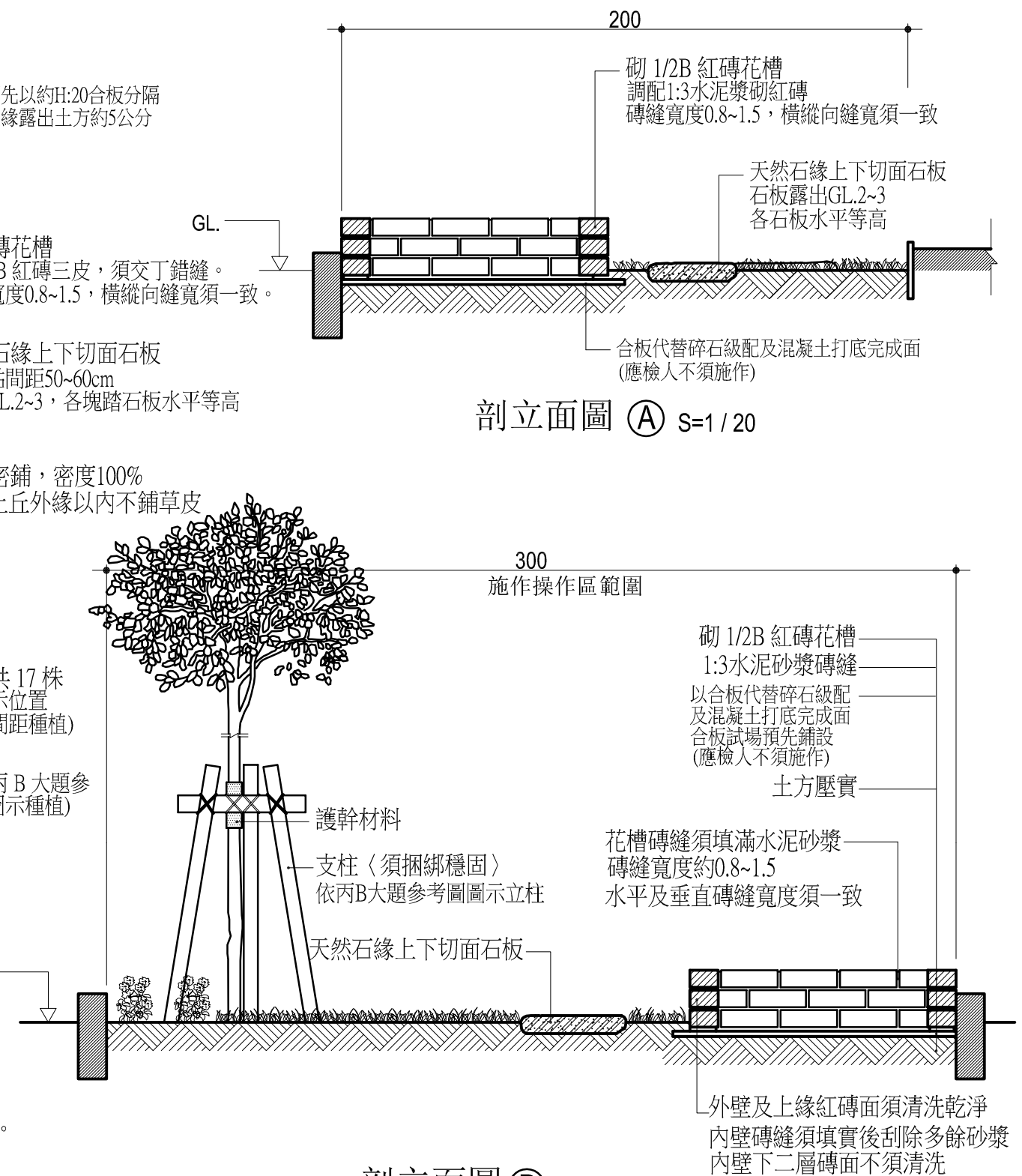
剖立面圖 (B) S=1/20
