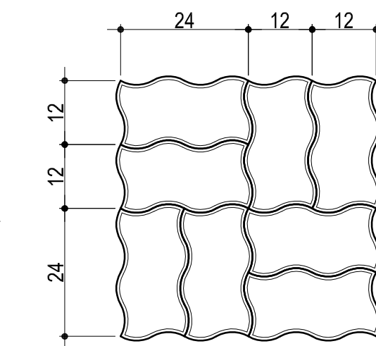
高壓水泥連鎖磚鋪設大樣示意圖 S=1 / 10
