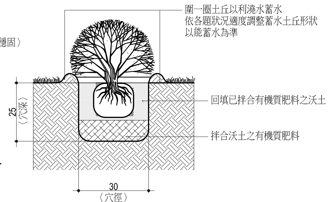
灌木種植剖面示意圖S=1 / 10
