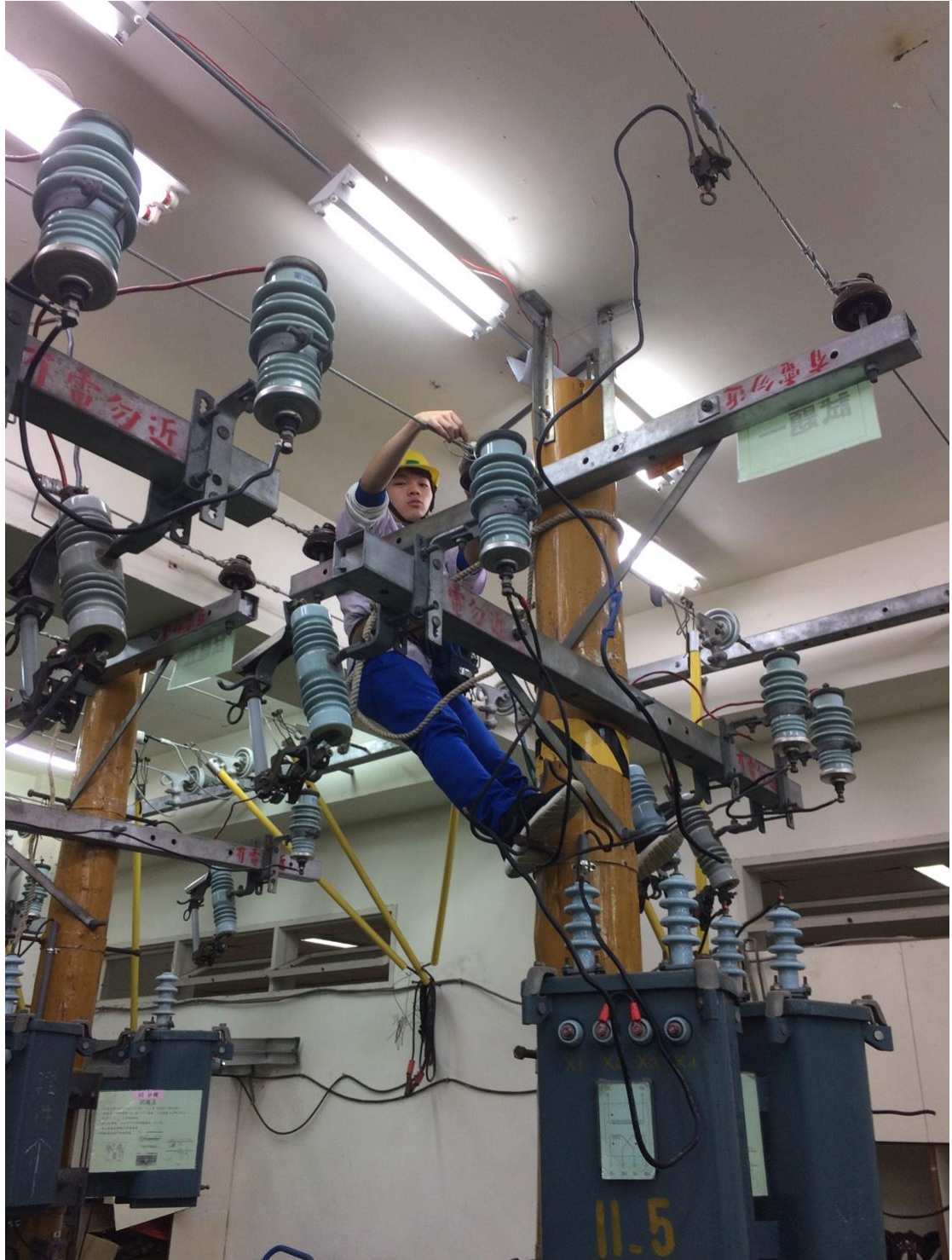
第三站 桿上變壓器實作(圖 1)
